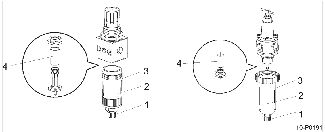
Abb. 22 Filterdruckminderer reinigen
