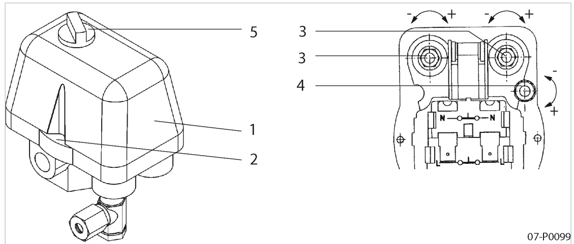
Abb. 8 Netzdruck einstellen
