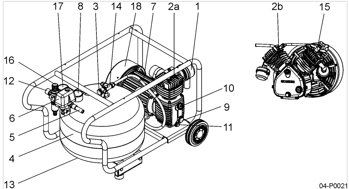
Abb. 2 Übersicht Maschine
