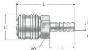
Schlauchanschluss
