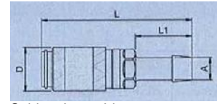
Schlauchanschluss
