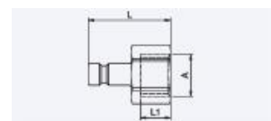
Innengewinde
