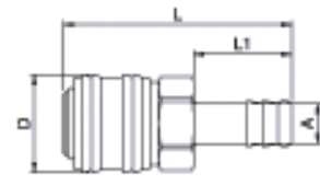
Schlauchtülle
