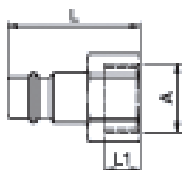
Nippel Innengewinde
