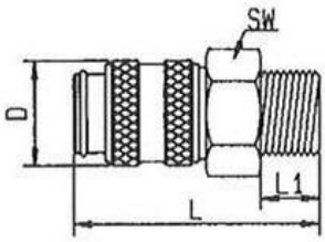
Außengewinde
