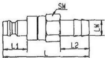
Tülle
