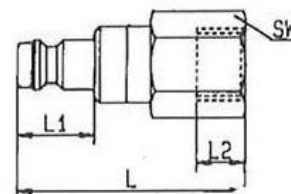
Nippel
