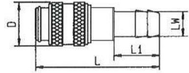
Schlauchanschluss
