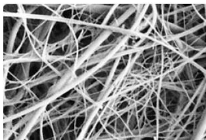
Mikroglasfaser
