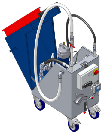
Seitenansicht 3-in-1-Hydraulikaggregat
